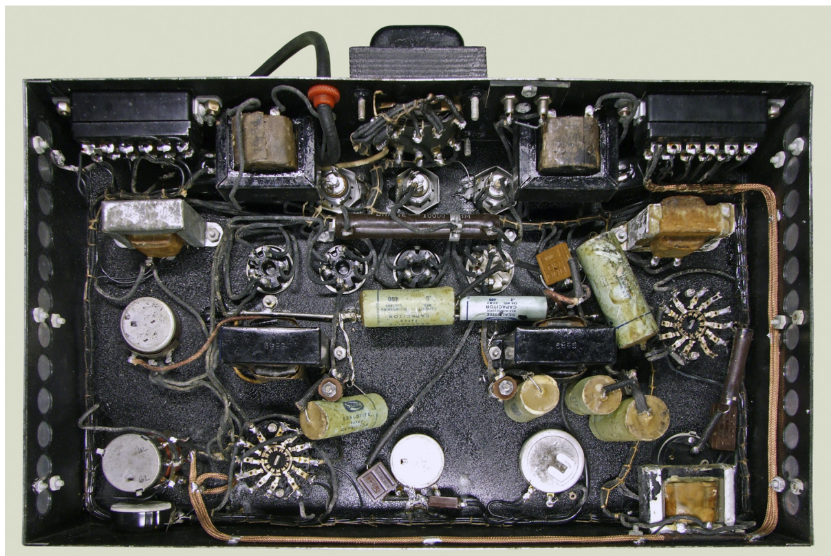
Vy under chassit visande radion med sina originalkomponenter.
